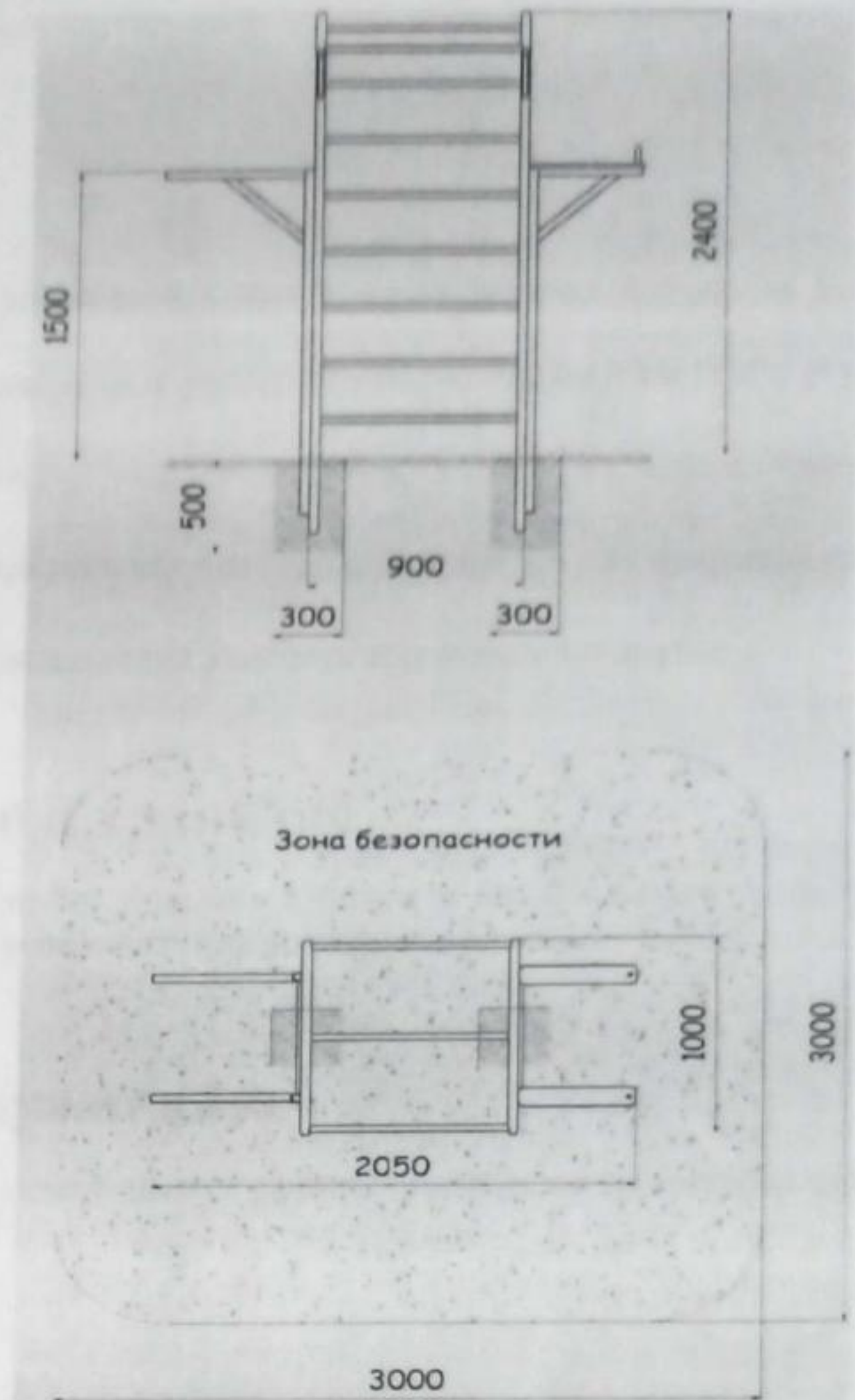
Рис.3 Основные размеры, схема расположения фундаментов и зона безопасности
